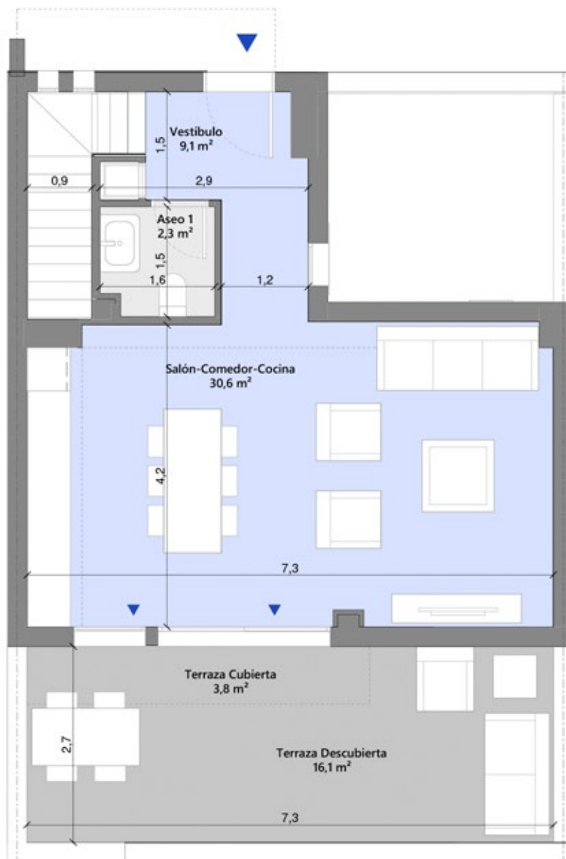
PLANTA BAJA
