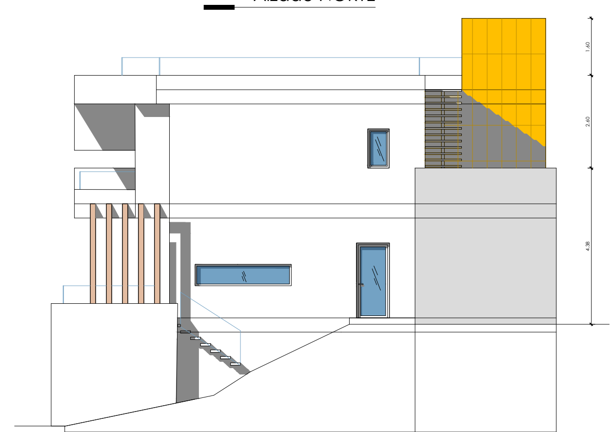
Alzado SUR
