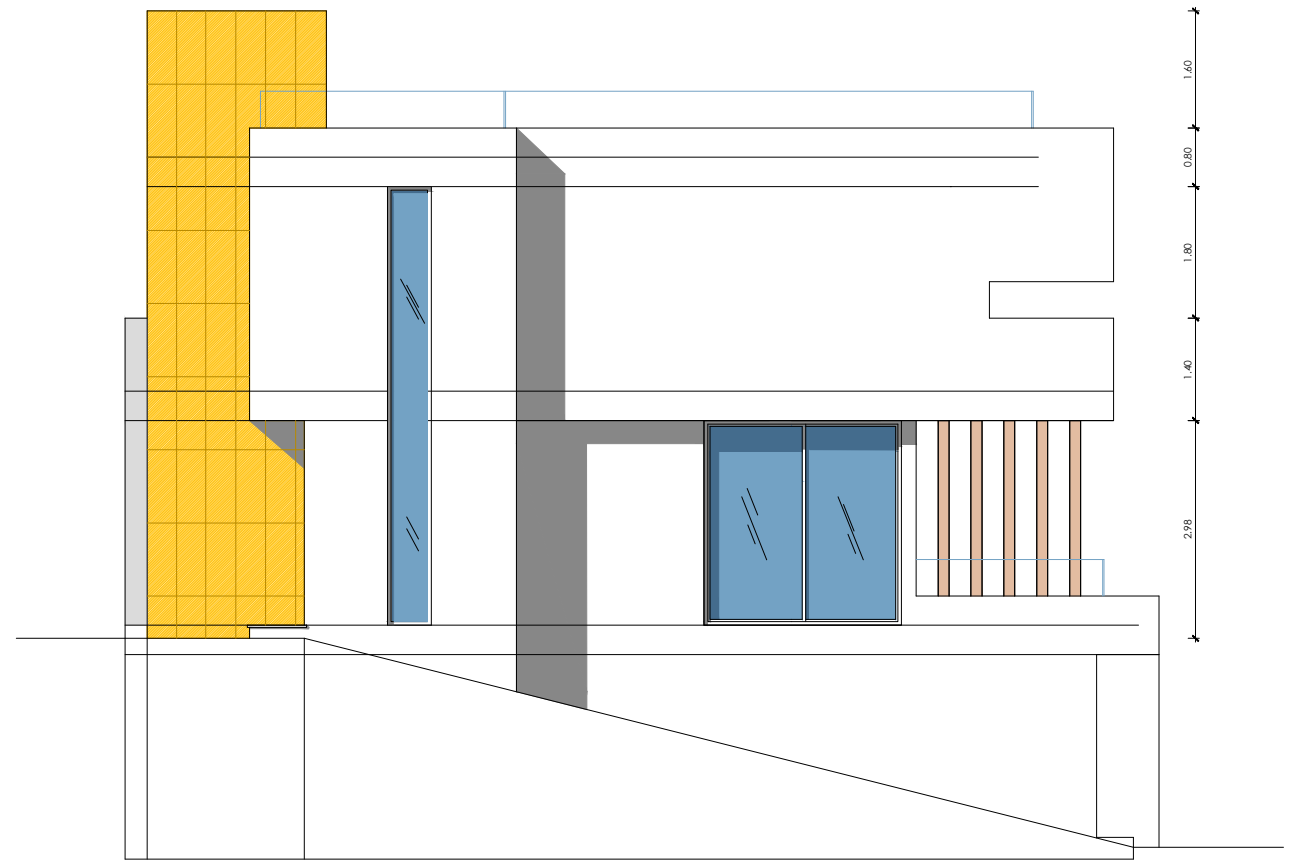
Alzado NORTE
