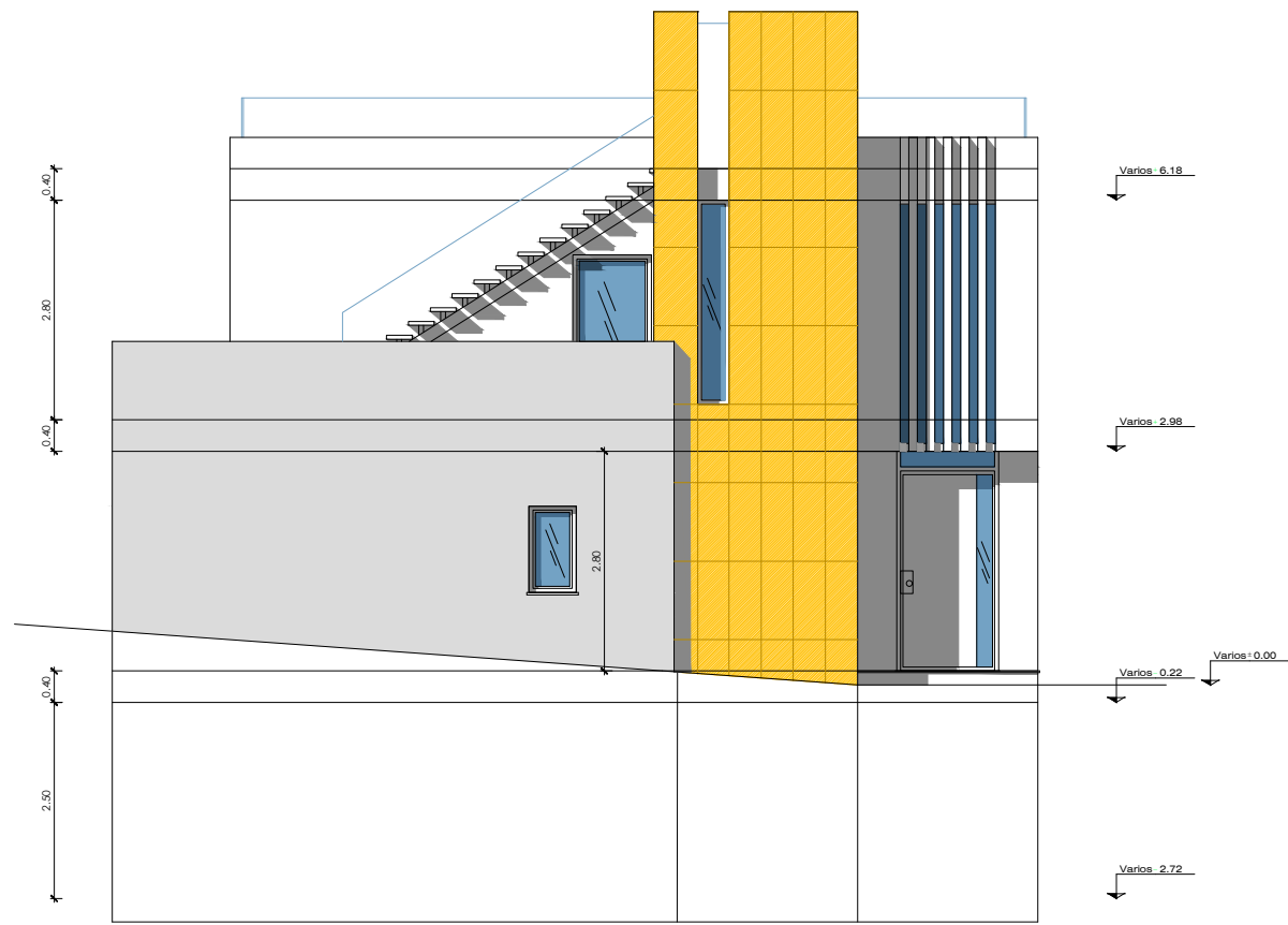
Alzado ESTE
