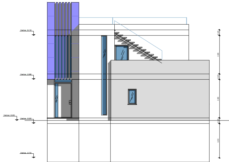
Alzado ESTE
