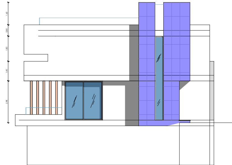
Alzado NORTE
