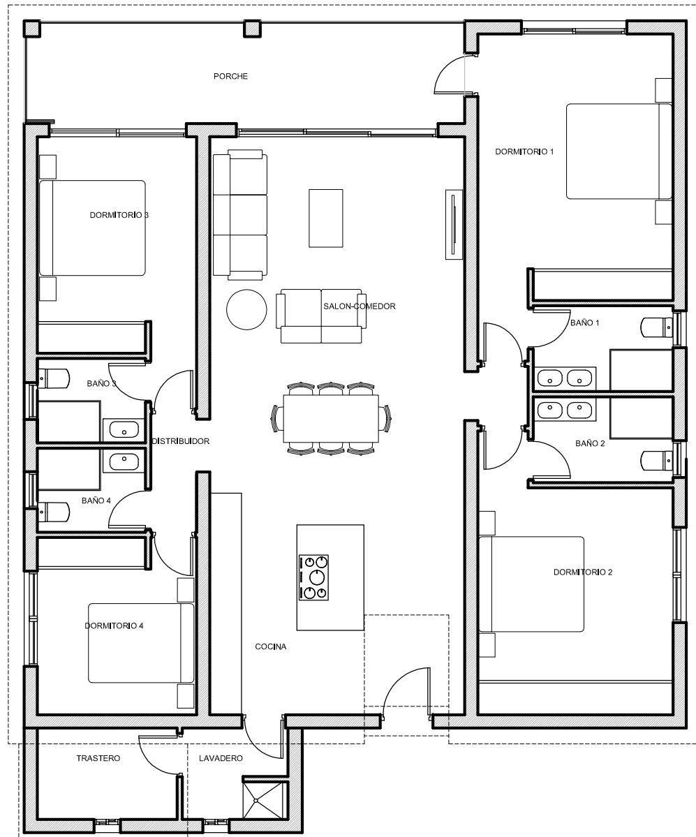
PLANTA DISTRIBUCION REFORMADO Esc: 1:100
