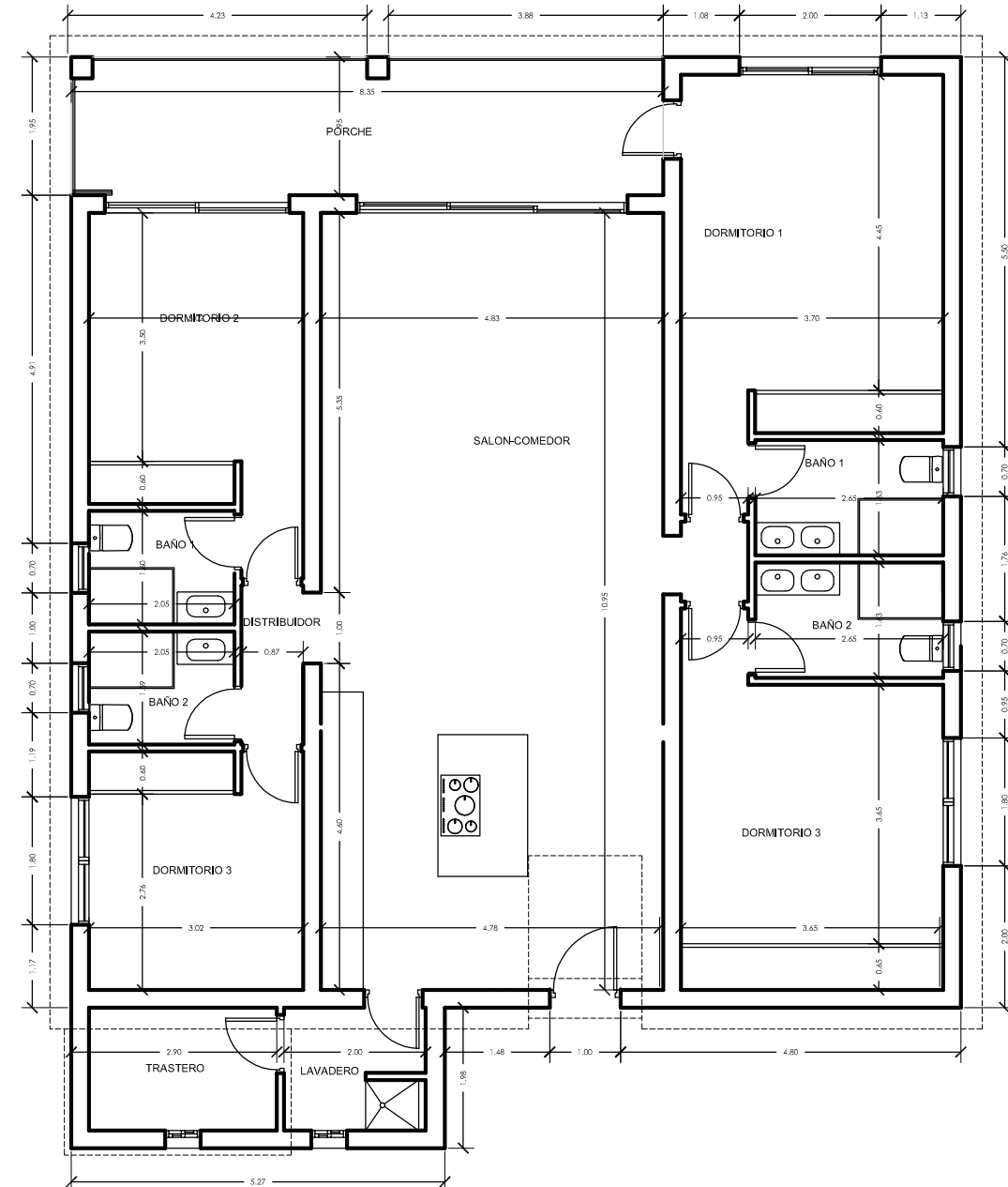
PLANTA ACOTADA REFORMADO Esc: 1:100
