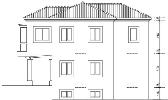
FACHADA NOROESTE
