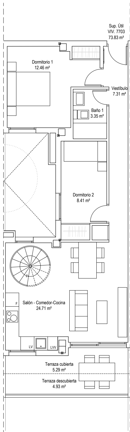
PLANTA INFERIOR
