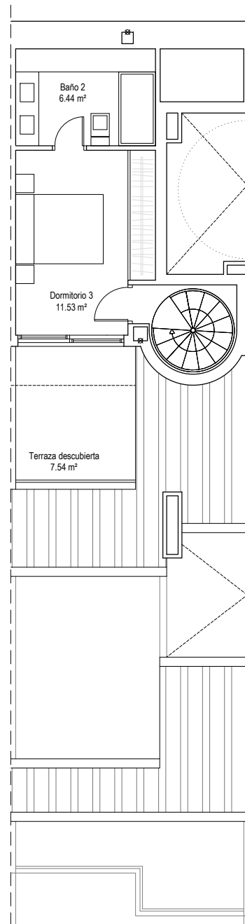
PLANTA SUPERIOR
