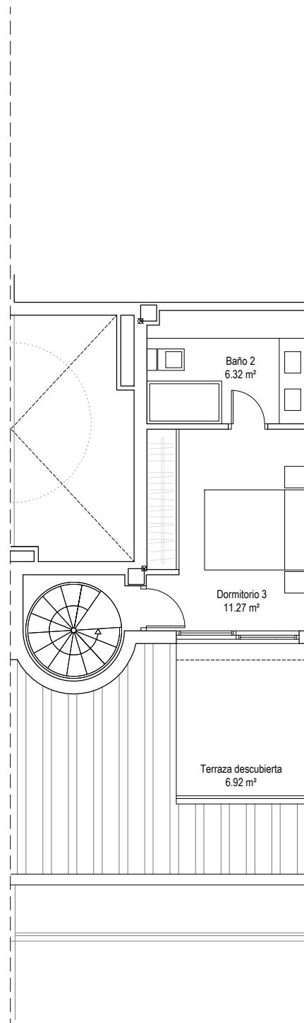
PLANTA SUPERIOR
