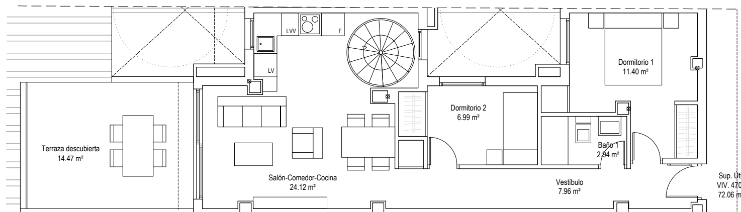
PLANTA INFERIOR
