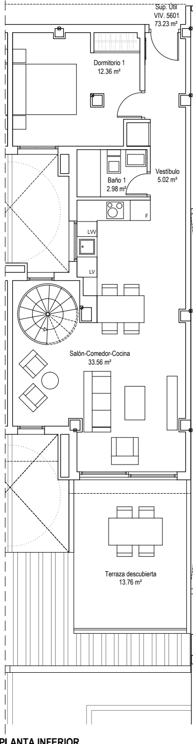
PLANTA INFERIOR
