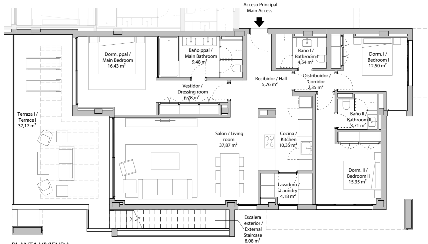
PLANTA VIVIENDA
