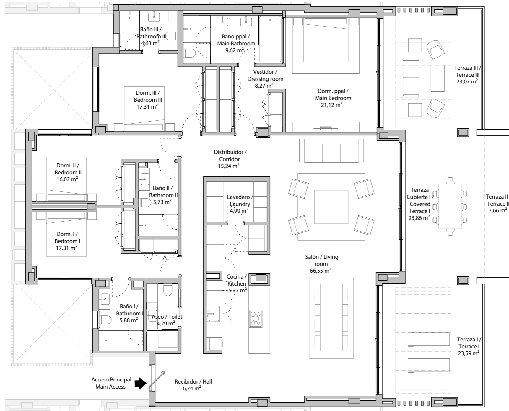
PLANTA VIVIENDA
