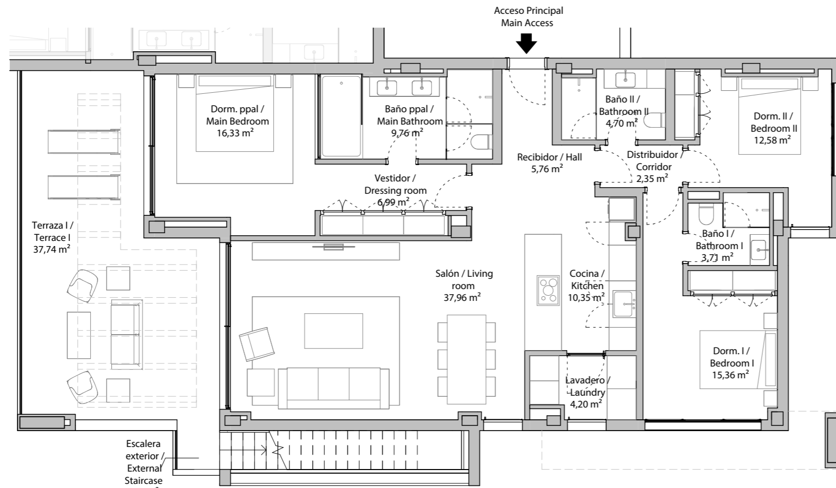
PLANTA VIVIENDA
