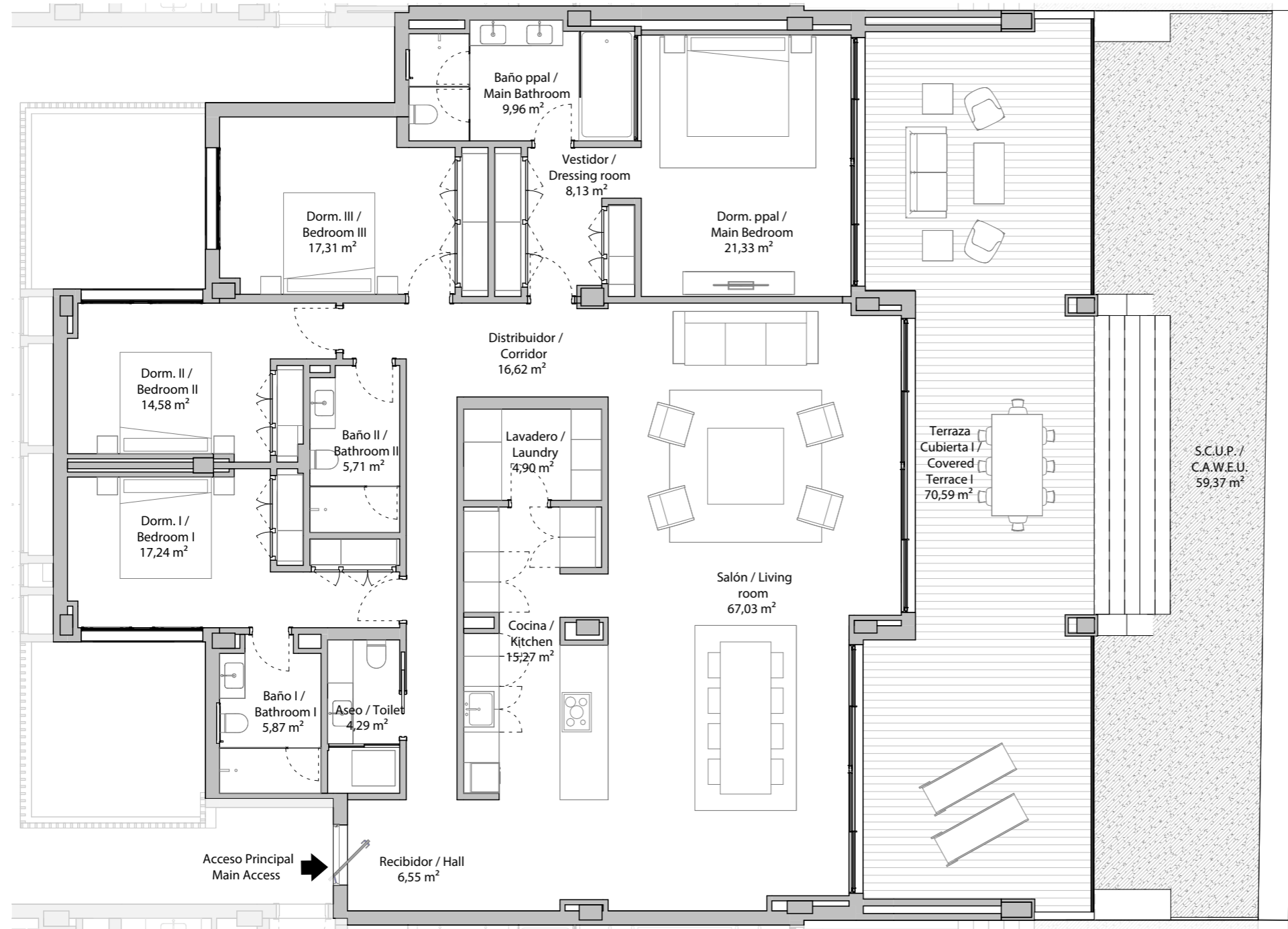
PLANTA VIVIENDA
