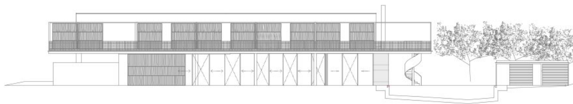
Alzado Oeste/West Elevation
