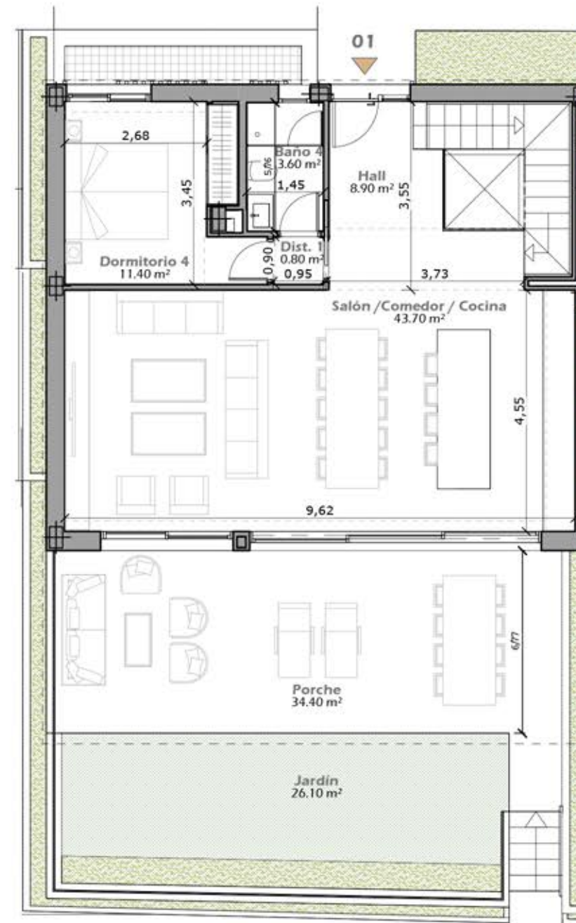
Planta Baja
