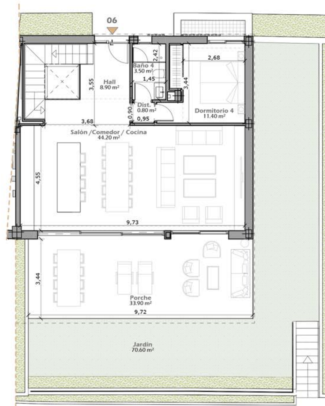
Planta Baja
