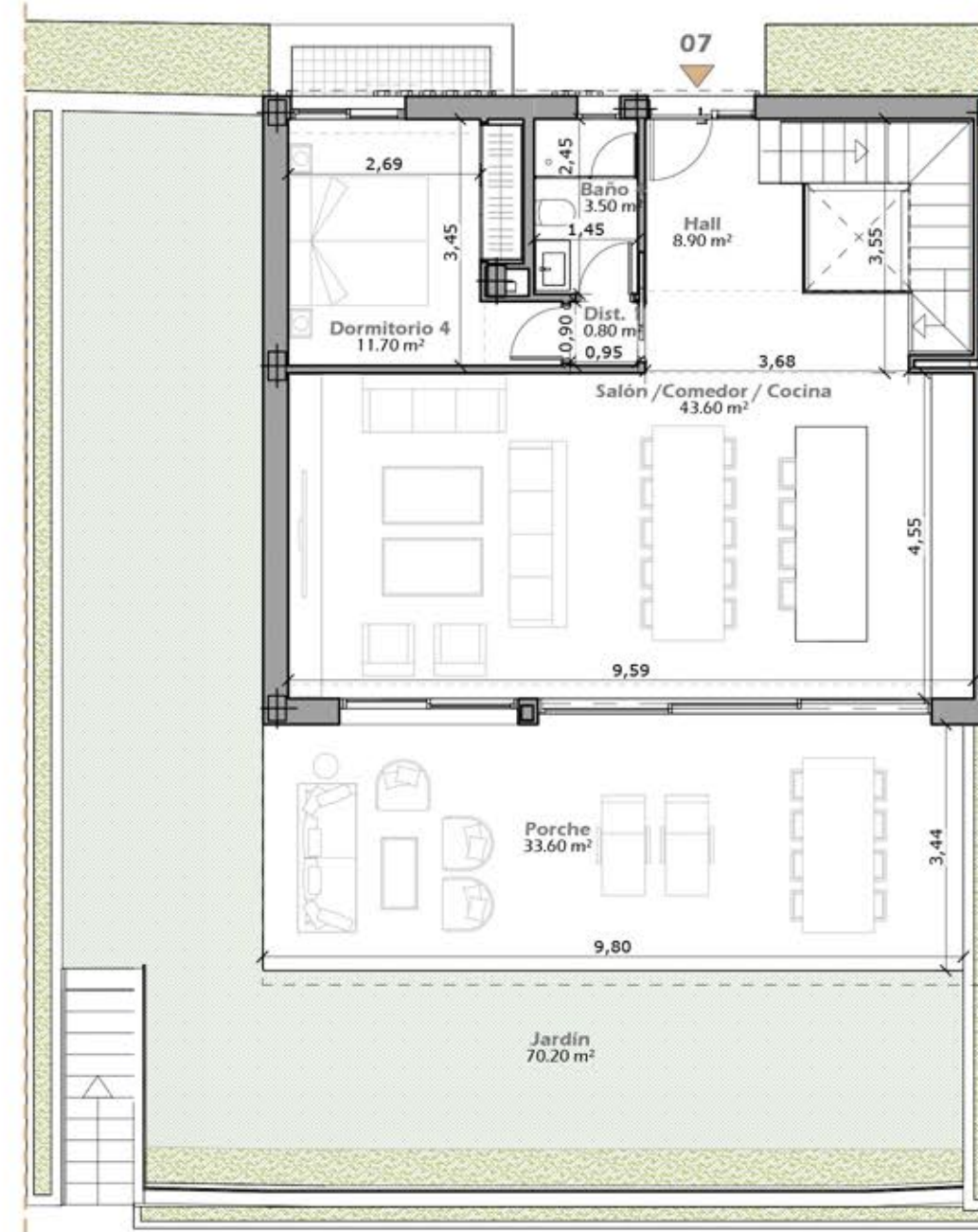
Planta Baja
