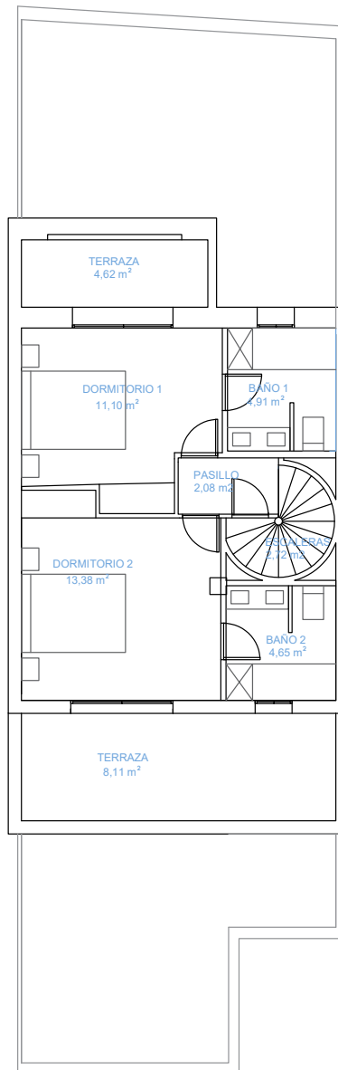
PLANTA PRIMERA
