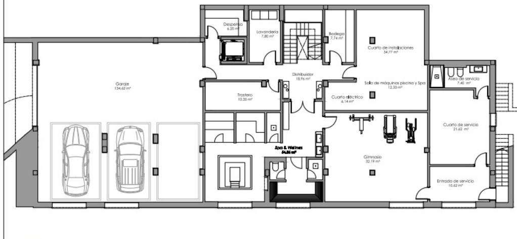
Planta sótano (Nivel 59.35)
