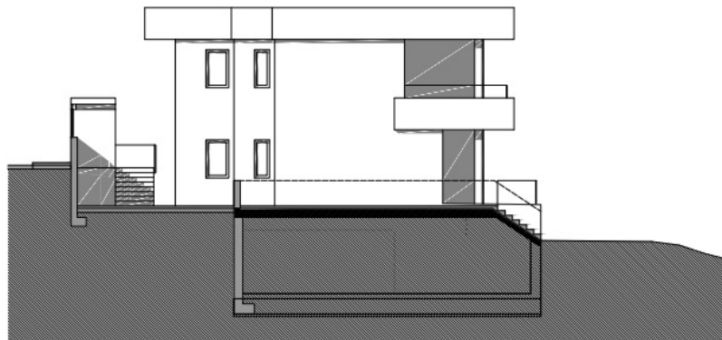
Alzado Sureste
