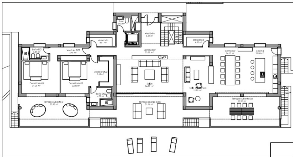
Planta baja (Nivel 62.90)
