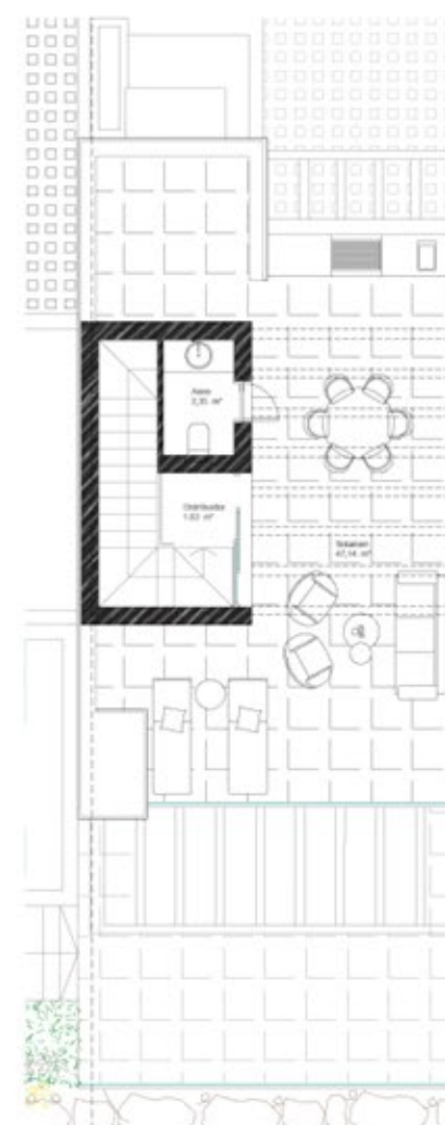
PLANTA 2
