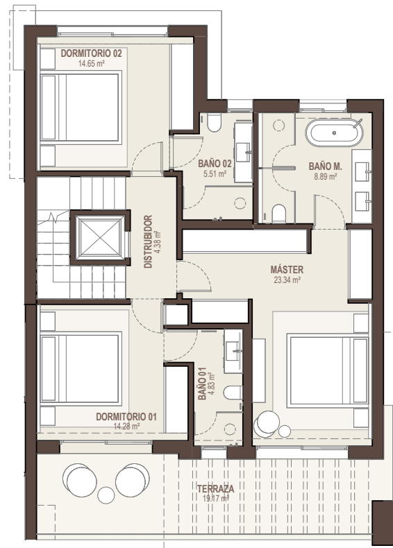
PLANTA ALTA 1 : 100
